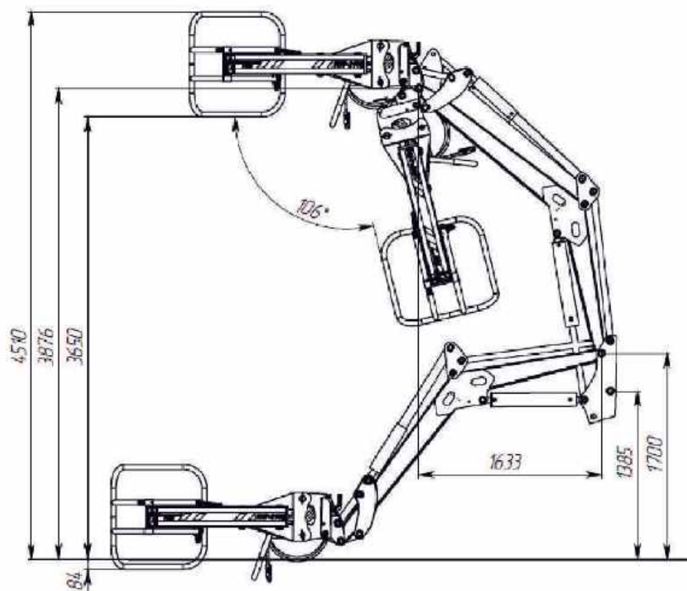
Кинематика погрузчика FRONTLIFT M с кантователем KHP-2100
