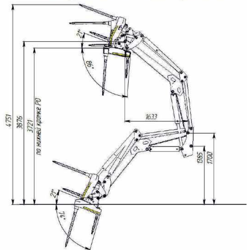
Кинематика погрузчика FRONTLIFT M EURO с вилами 3х зубыми ВЛ3-081EURO
