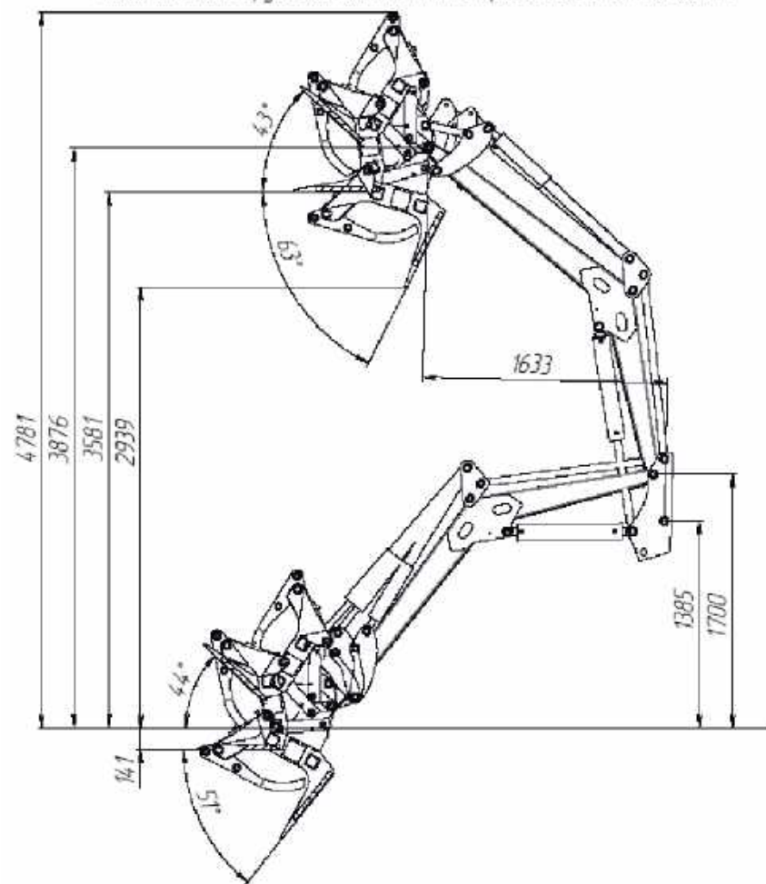
Кинематика погрузчика FRONTLIFT М с Бревнозахватом БЗ-081 FL
