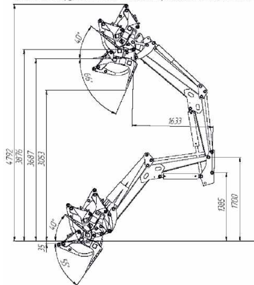
Кинематика погрузчика FRONTLIFT М EURO с Бревнозахватом БЗ-081 EURO
