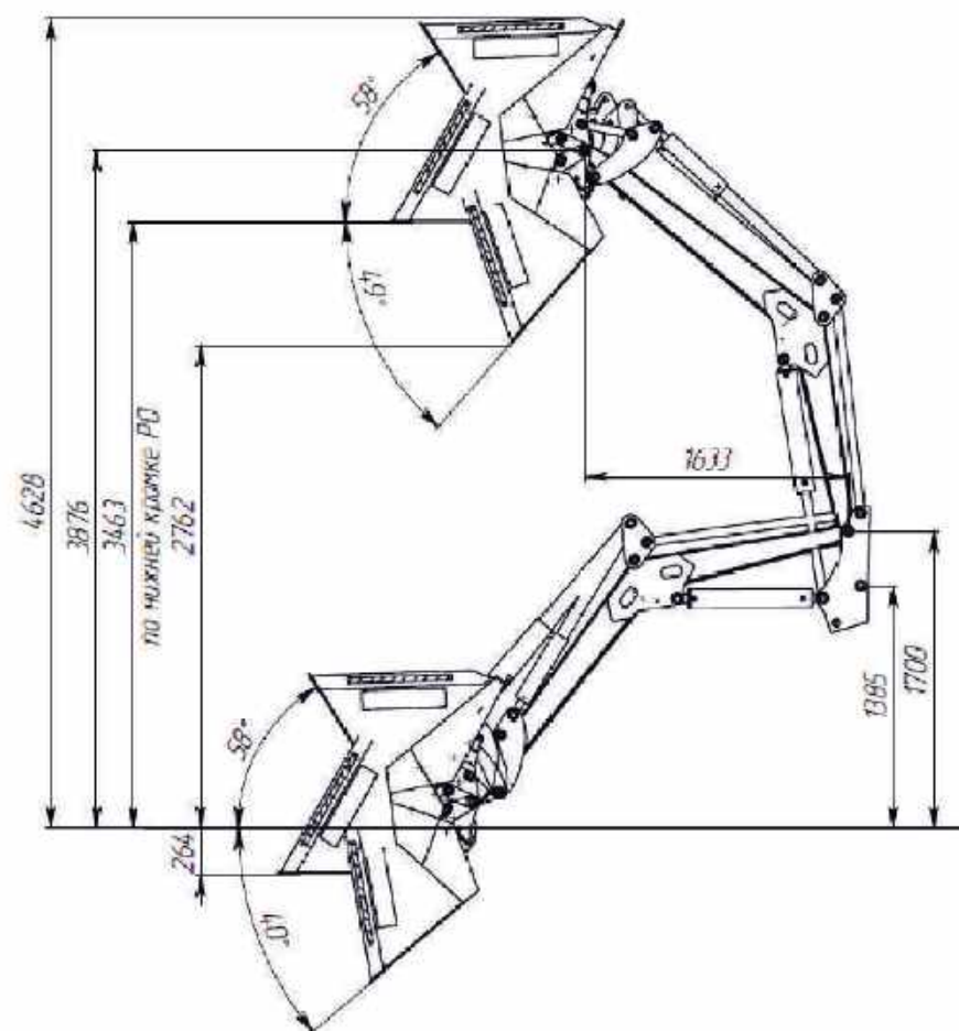
Кинематика погрузчика FRONTLIFT М EURO с ковшом КШ-011EURO
