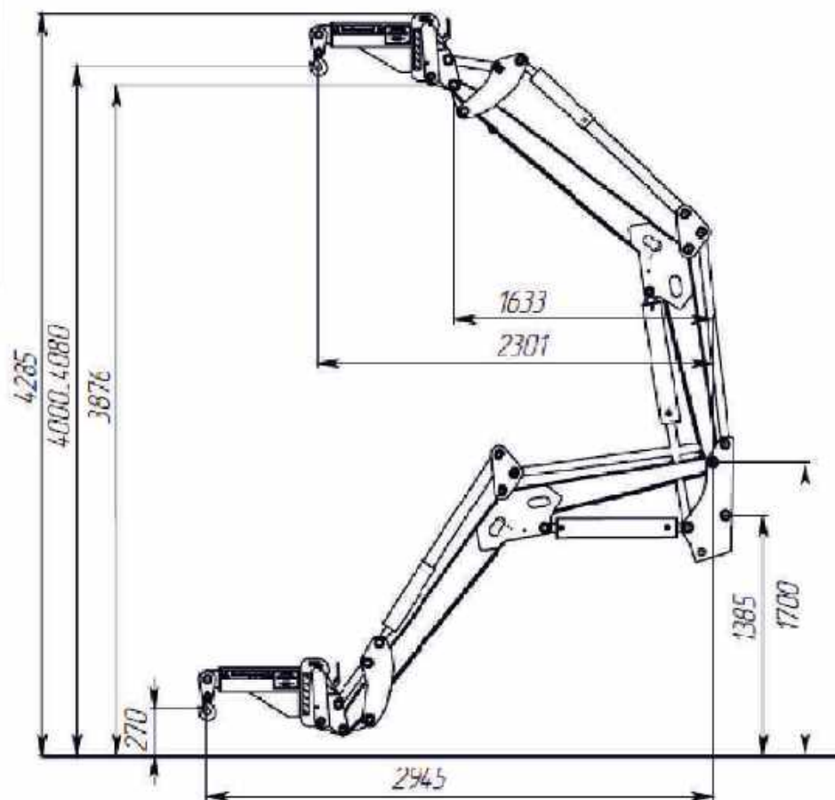
Кинематика погрузчика FRONTLIFT М с грузоподъемным устройством ГПУ-081FL
