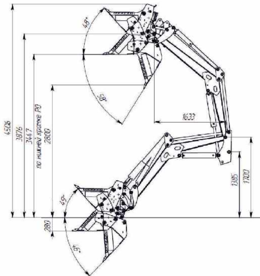
Кинематика погрузчика FRONTLIFT М с ковшом КШЧ-07FL
