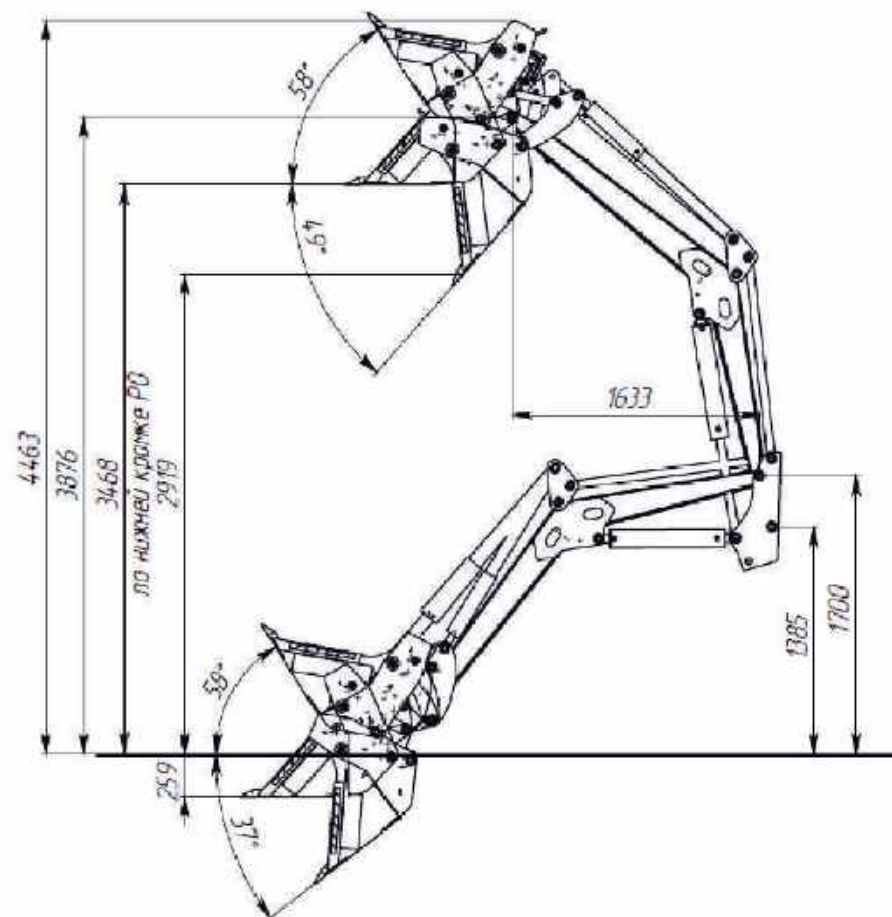
Кинематика погрузчика FRONTLIFT М EURO с ковшом КШЧ-07EURO
