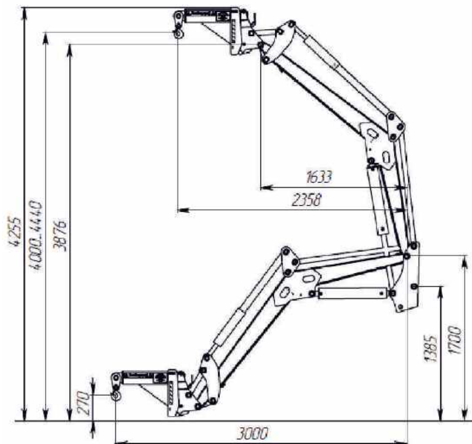
Кинематика погрузчика FRONTLIFT М EURO с грузоподъемным устройством ГПУ-081EURO
