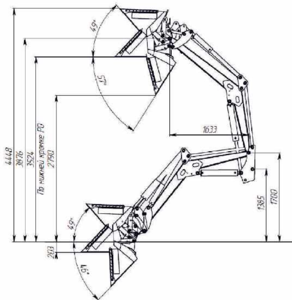
Кинематика погрузчика FRONTLIFT М с ковшом КШ-06FL
