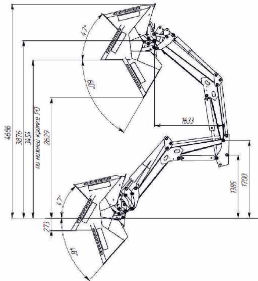
Кинематика погрузчика FRONTLIFT М с ковшом КШ-011FL
