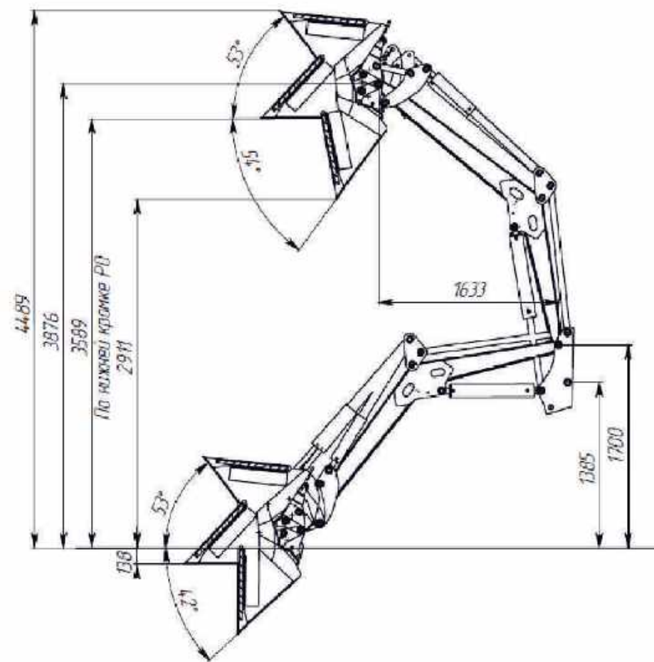
Кинематика погрузчика FRONTLIFT М EURO с ковшом КШ-06EURO
